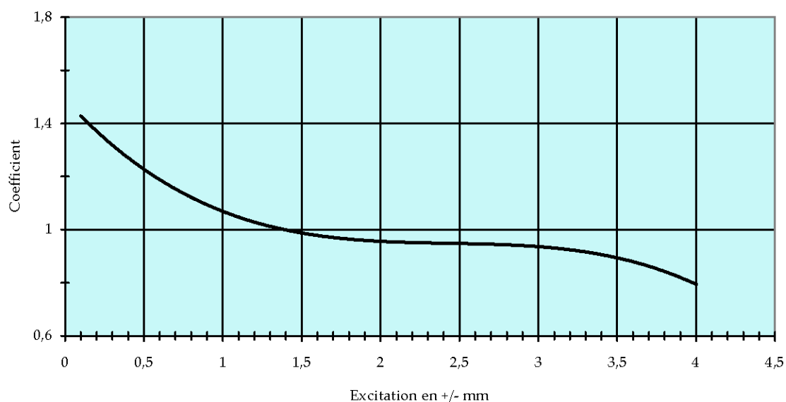
Courbe typique de rigidification
